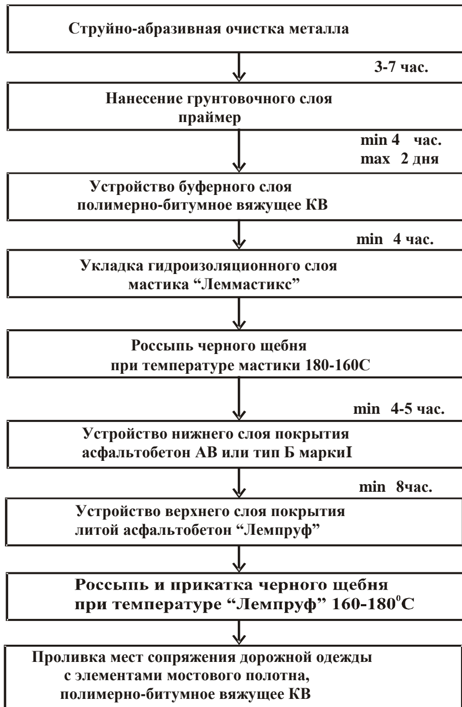
Рисунок 12 - Схема технологического процесса устройства конструкции дорожной одежды на ортотропной плите проезжей части при устройстве гидроизоляционного слоя мастики «Леммастикс»
