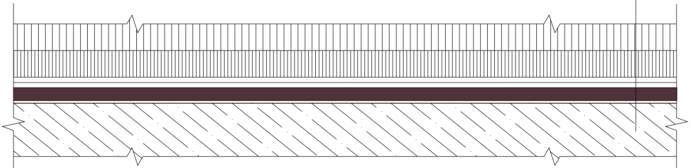
Рисунок 2 - Гидроизоляция ортотропной плиты мостового сооружения.
